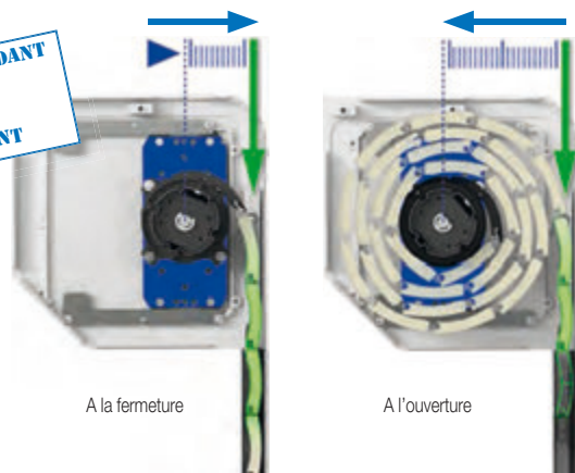
Déplacement du chariot
