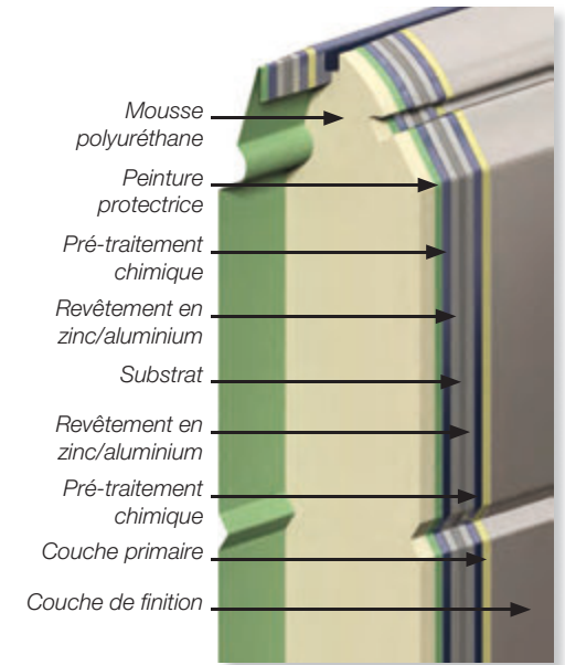
Profil panneau isolé
