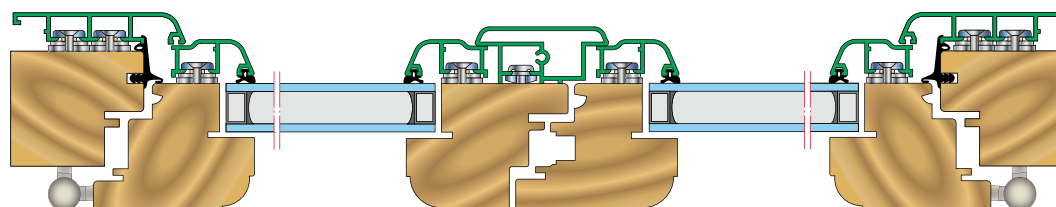
coupe horizontale d'une fenêtre bois - aluminium 2 vantaux
