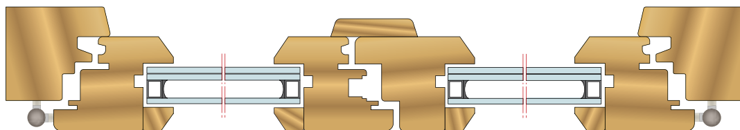
coupe d'une fenêtre bois à 2 vantaux
