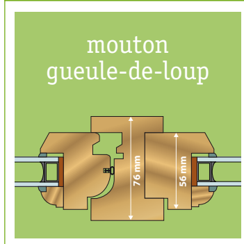
coupe d'une fenêtre bois à 2 vantaux
