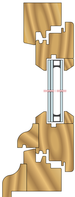
coupe d'une fenêtre bois à 2 vantaux
