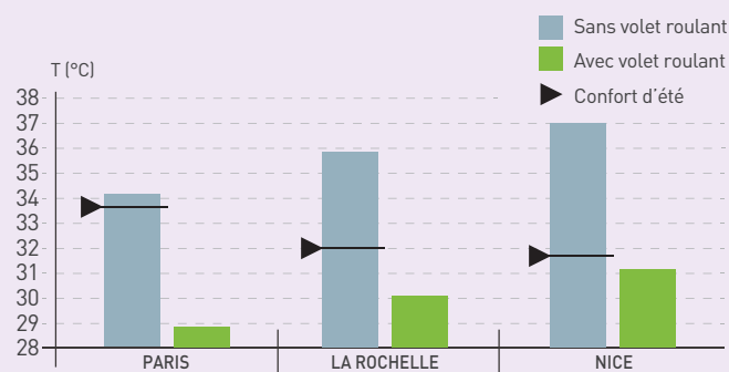
Impact du volet roulant ( \Delta R ) sur la température intérieure d'une maison (double vitrage)
